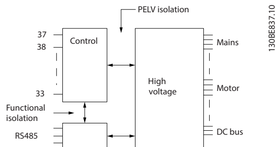
Ilustración 9.1 Aislamiento galvánico
